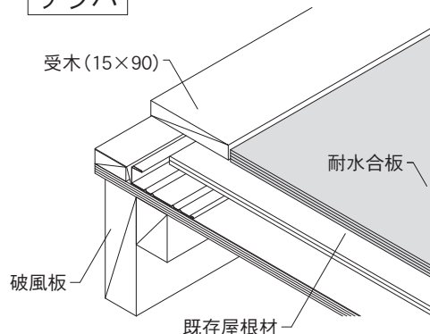
ケラバ
