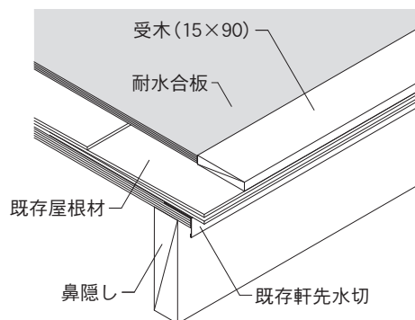
軒先
