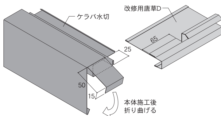
施工手順 1) <改修用唐草Dを使用する場合>
